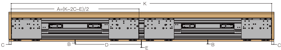
四门柜体参数图 Four doors cabinet parameters
