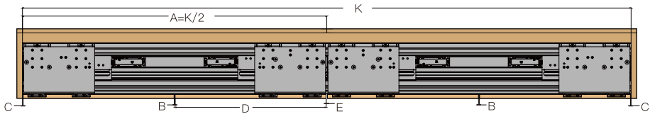
四门柜体参数图 Four doors cabinet parameters
